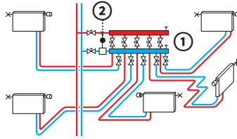
die Etagenweise Verteilung heat distribution to multiple storeys توزیع أحادي المرحلة توزیع گرما به شکل مسطح
