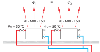
das Zweirohrsystem two-pipe ((central-)heating) system نظام الأنبوب الثنائي سیستم دولوله ای
