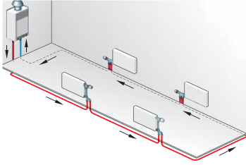
die Etagenheizung single-storey heating system نظام تدفئة من طابق واحد گرمایش از کف
