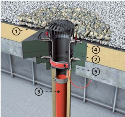
④ der Klemmflansch clamping ring
