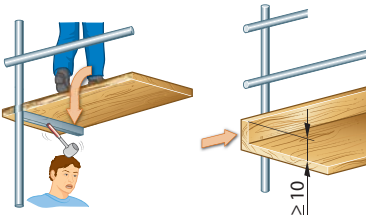
das Bordbrett toe board معرضة سفلية تخته دار بست
