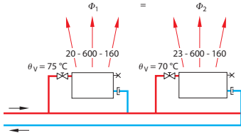
das Einrohrsystem single-pipe ((central-)heating) system نظام الأنبوب الأحادي سیستم یک لوله ای
