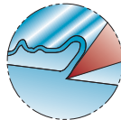
der Fließspan continuous chip
